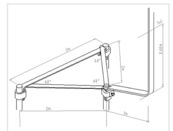
Ejemplo de puesta a tierra
