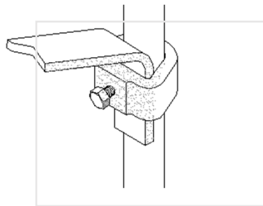
Entregado con un tornillo M10 latón
