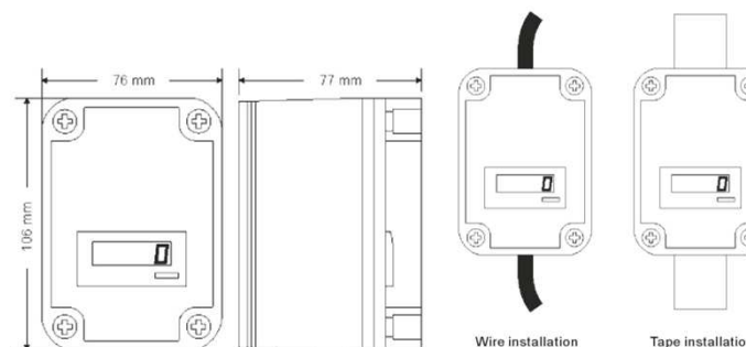
Esquema dimensional
